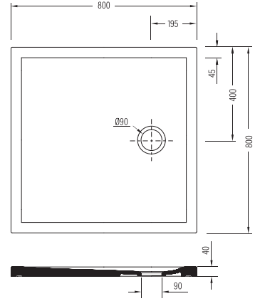
DUŞ TEKNESİ BEYAZ TPTD00002F02W5000 80X80 CM
