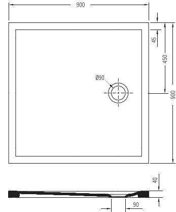
DUŞ TEKNESİ BEYAZ TPTD00003F02W5000 90X90 CM
