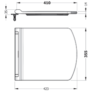
SALVO MONOSLIM UF/ DUROPLAST AB YAVAŞ KAPANIR KOLAY TAK ÇIKAR KLOZET KAPAĞI SVMU11W5W5HB0
