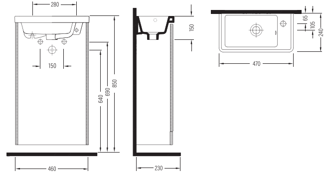
MOBİLYA UYUMLU LAVABO SAĞDAN BATARYA DELİKLİ KSLKR47B1FD1W5000 470x240mm
