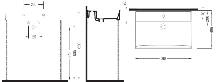
MOBİLYA UYUMLU TEZGAH ÜSTÜ LAVABO BATARYA DELİKLİ MSLG080B1FD1W5000 810x465mm
