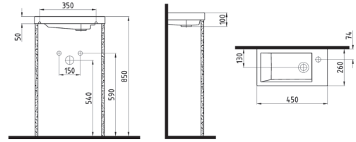
MOBİLYA UYUMLU LAVABO SAĞDAN BATARYA DELİKLİ INLK04501FD1W5000 450mm
