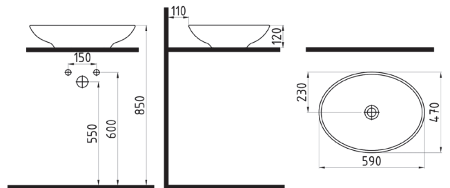
TEZGAH ÜSTÜ LAVABO HRLG05901FDOW5000 590x470mm
