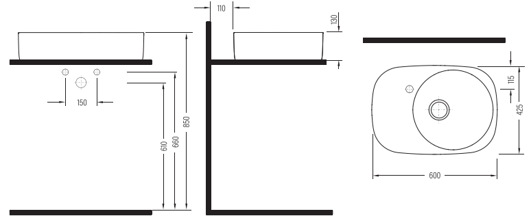
TEZGAH ÜSTÜ LAVABO SOL TARAFTAN BATARYA DELİKLİ SQLGL6001FD1W5000 600x425 mm
