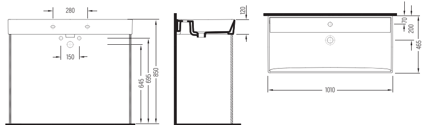
MOBİLYA UYUMLU TEZGAH ÜSTÜ LAVABO BATARYA DELİKLİ MSLG10001FD1W5000 1010x465mm
