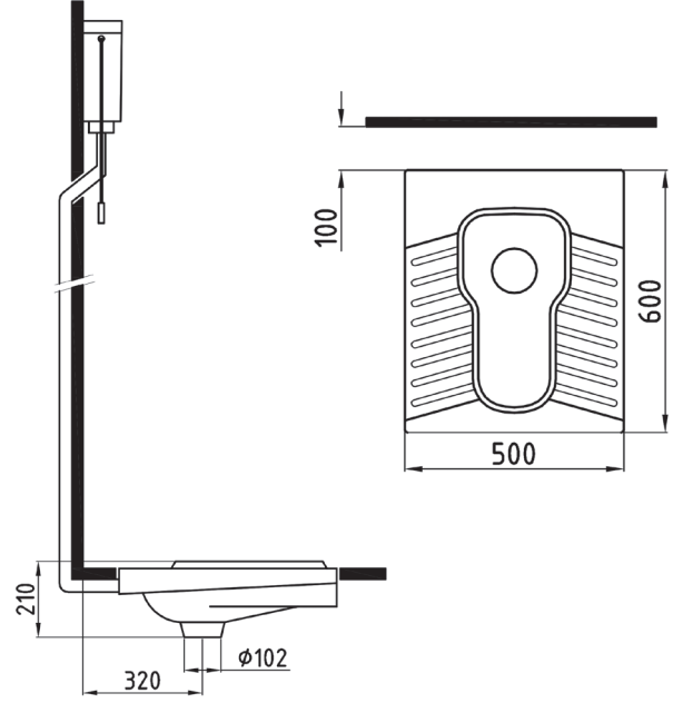
TEK PARÇA HELA TAŞI ARKADAN SU GİRİŞLİ TPHT05002VSAW5000 500x600mm
