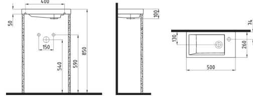
MOBİLYA UYUMLU LAVABO SAĞDAN BATARYA DELİKLİ INLK05001FD1W5000 500mm
