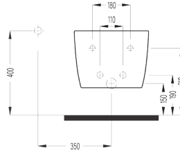
ASMA BİDE SOBA05201VD1W5000 520x355 mm
