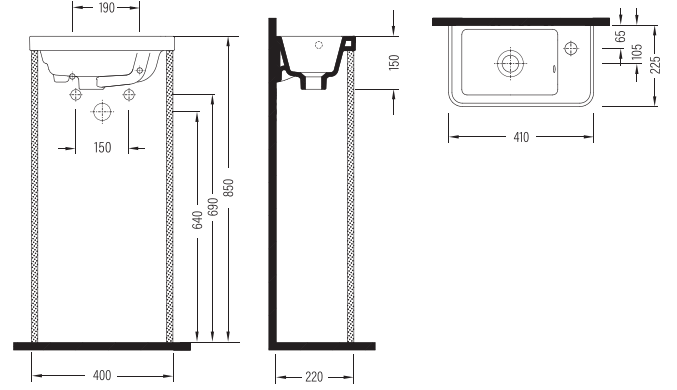
MOBİLYA UYUMLU LAVABO SAĞDAN BATARYA DELİKLİ KSLKR41B1FD1W5000 410x225mm
