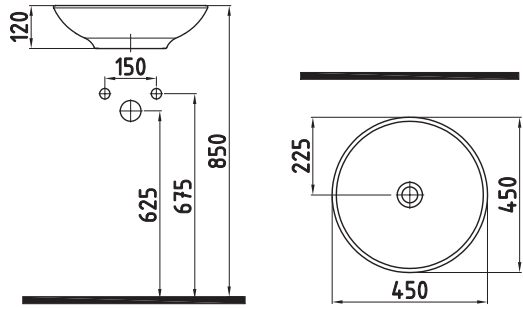
TEZGAH ÜSTÜ LAVABO HRLG04501FDOW5000 Ø450mm
