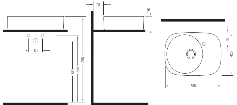
TEZGAH ÜSTÜ LAVABO SAĞ TARAFTAN BATARYA DELİKLİ SQLGR6001FD1W5000 600x425 mm
