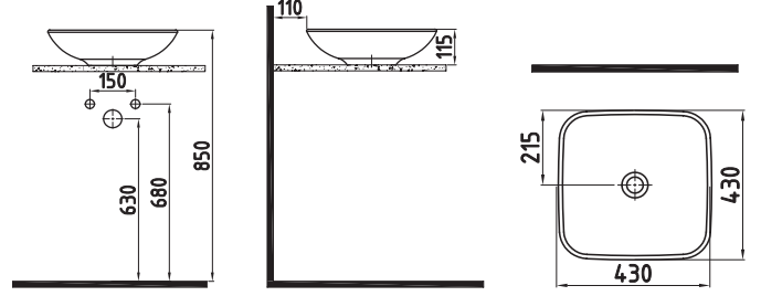
TEZGAH ÜSTÜ LAVABO HRLG04301FDOW5000 430x430mm
