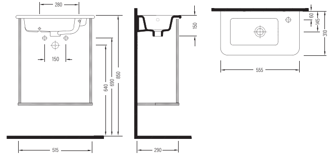
MOBİLYA UYUMLU LAVABO SAĞDAN BATARYA DELİKLİ KSLKR55B1FD1W5000 555x310mm
