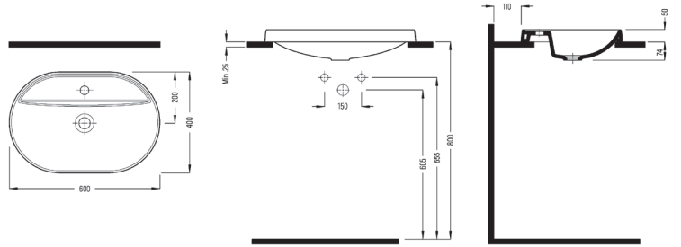
TEZGAH ÜSTÜ GÖMME LAVABO BATARYA DELİKLİ SOLU06001FD1W5000 600x400 mm
