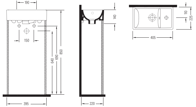
TEZGAH ÜSTÜ LAVABO SAĞDAN BATARYA DELİKLİ KSLGR40B1FD1W5000 405x225mm
