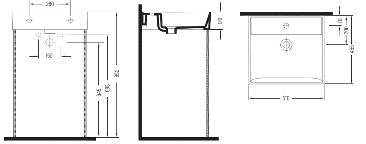
MOBİLYA UYUMLU TEZGAH ÜSTÜ LAVABO BATARYA DELİKLİ MSLG050B1FD1W5000 510x465mm
