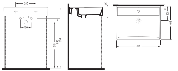
MOBİLYA UYUMLU TEZGAH ÜSTÜ LAVABO BATARYA DELİKLİ MSLG060B1FD1W5000 610x465mm
