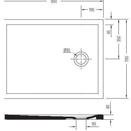
DUŞ TEKNESİ BEYAZ TPTD00001F02W5000 70X90 CM
