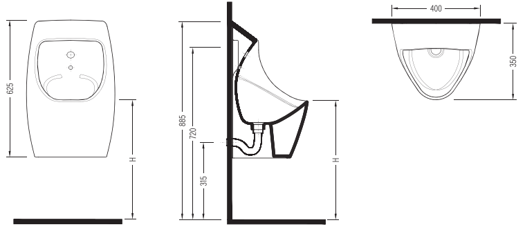
HARMONY PİSUVAR ARKADAN SU GİRİŞLİ ELEKTRİKLİ / PİLLİ HRPS06205VSAW5000 400x350mm
