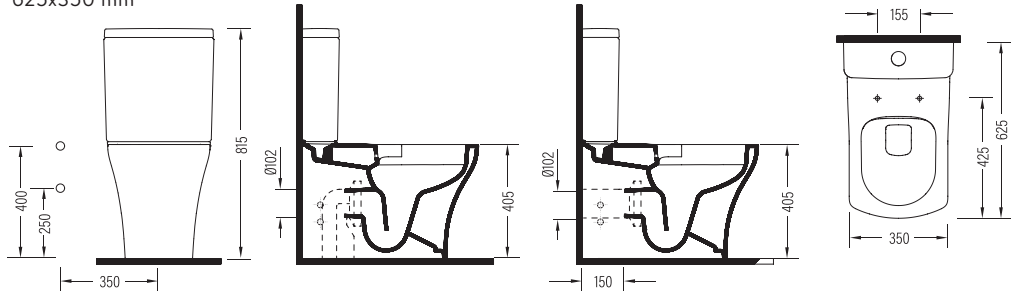
KÖŞELİ DUVARA SIFIR KLOZET TAKIMI NO-RIM RSKD063N1VP1W5000 625x350 mm
