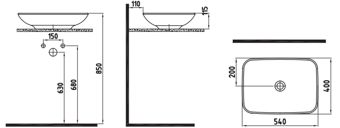
TEZGAH ÜSTÜ LAVABO HRLG05401FDOW5000 540x400mm
